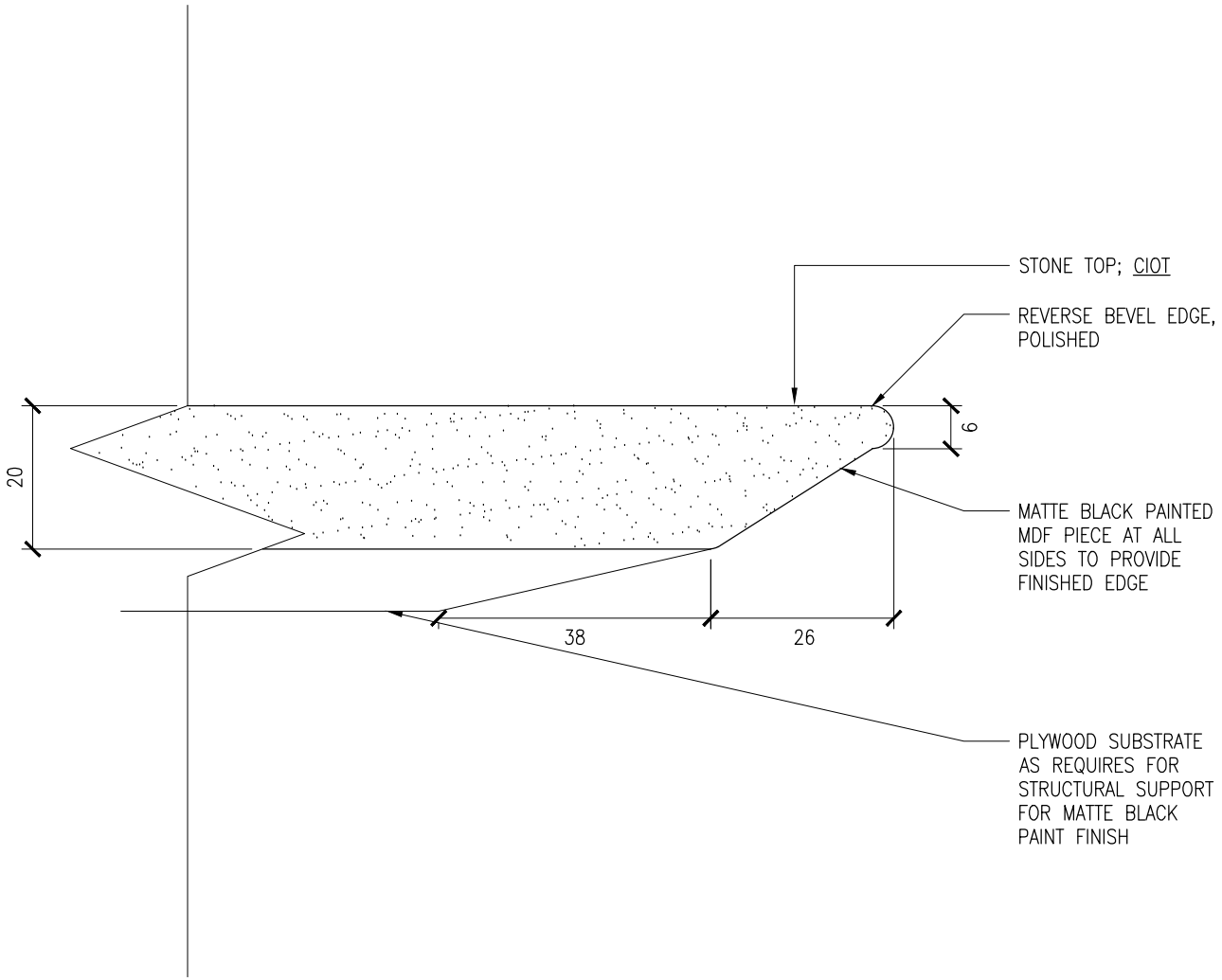
1 TABLE EDGE DETAIL D3.11.1 SCALE 1:1
