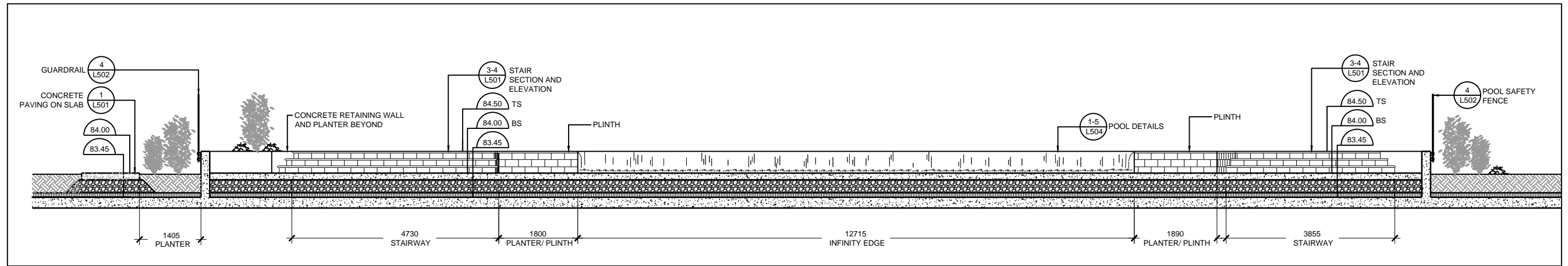
1 AMENITY TERRACE: INFINITY EDGE ELEVATION SCALE: 1 : 50
